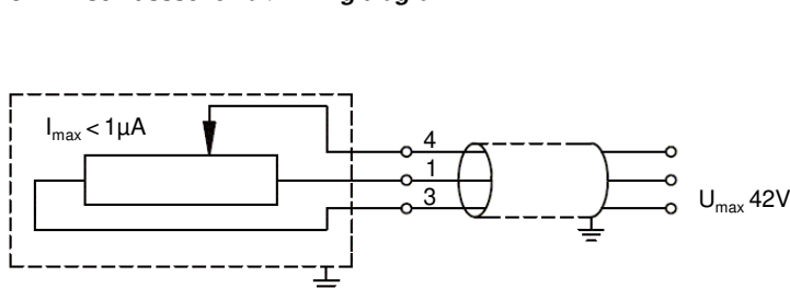
Dargestellte Belegung für ausfahrende Schubstange Shown configuration for extending rod
