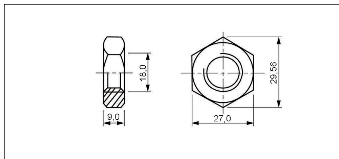
安装螺母 ISO 8675
