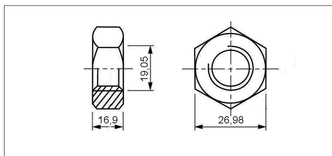
安装螺母 DIN 934
