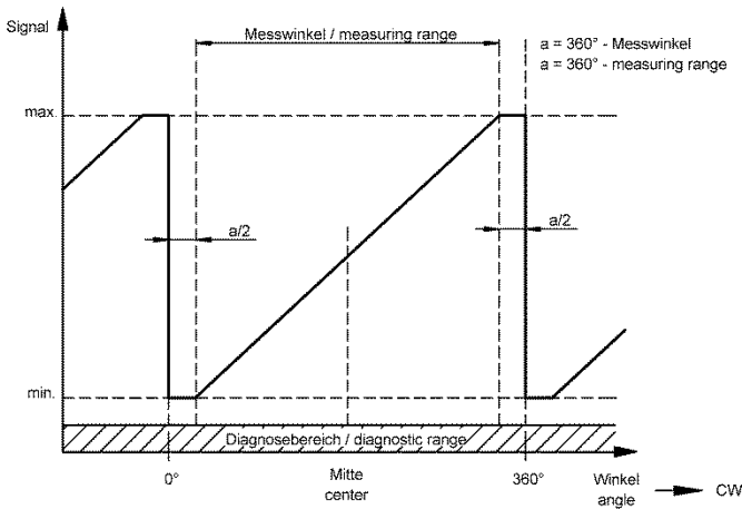
Einkanalig / single
