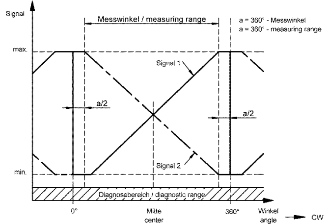
Mehrkanalig / redundant
